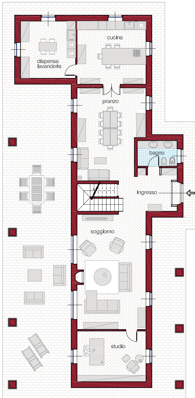
Planimetria Progetto di Massima - Piano Terreno -
