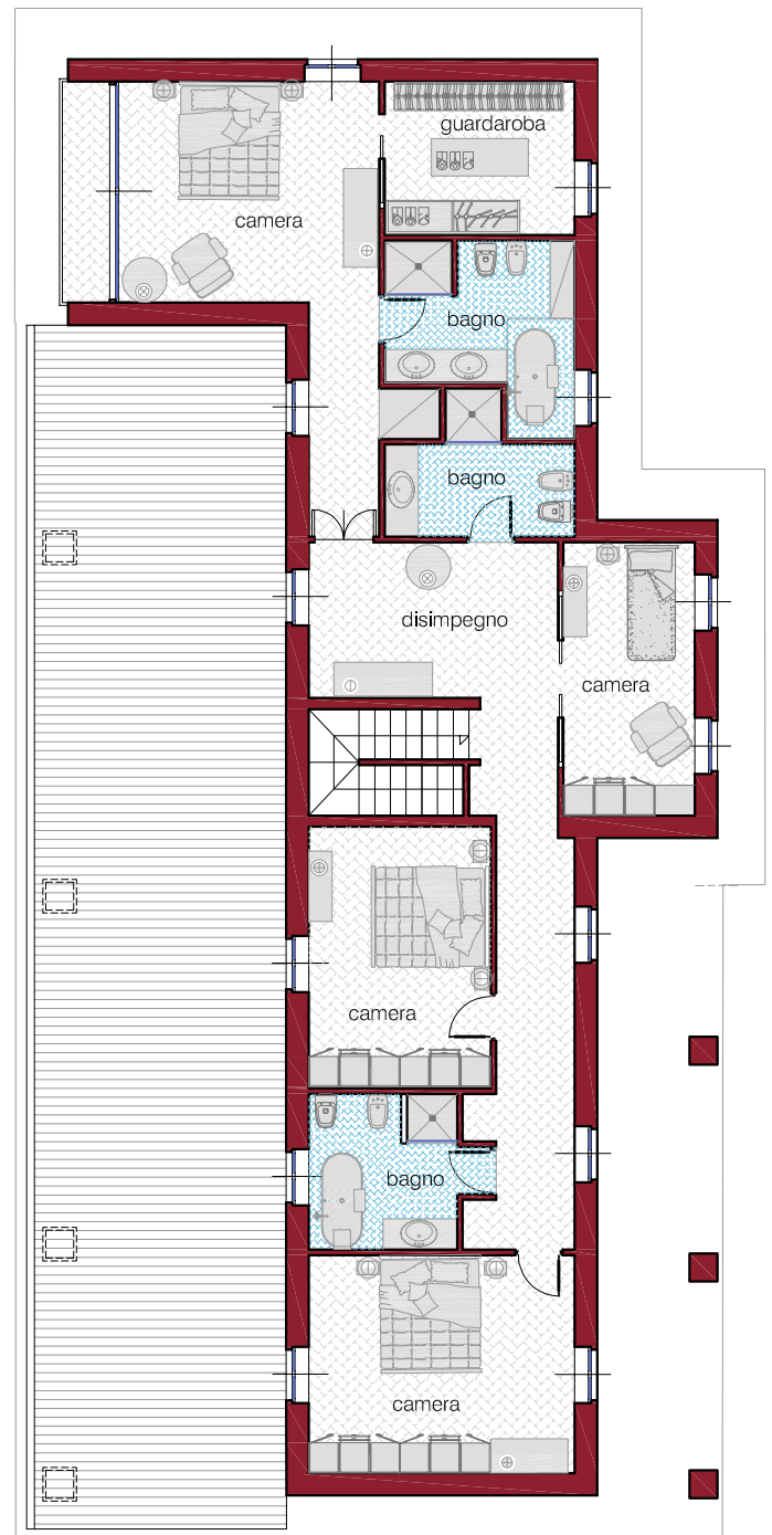
Planimetria Progetto di Massima - Piano Primo -
